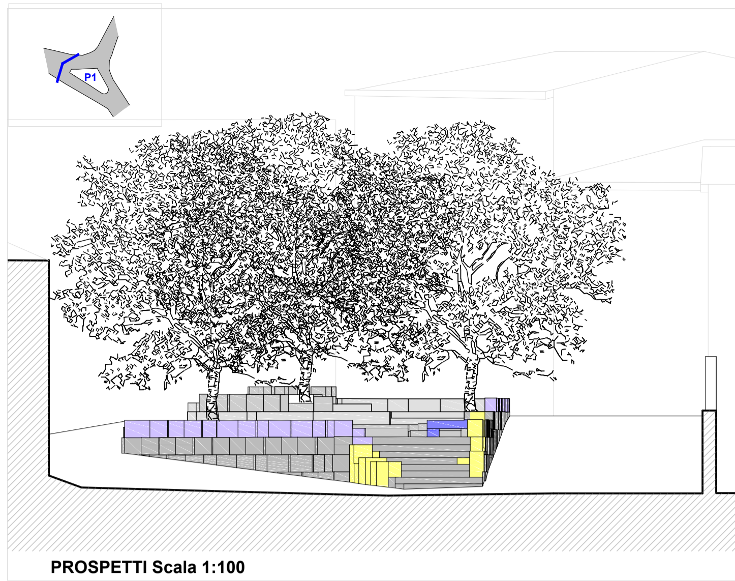
PROSPETTI Scala 1:100
